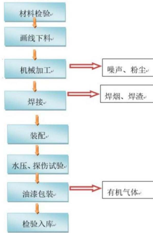
图3-2 主要生产工艺流程图
